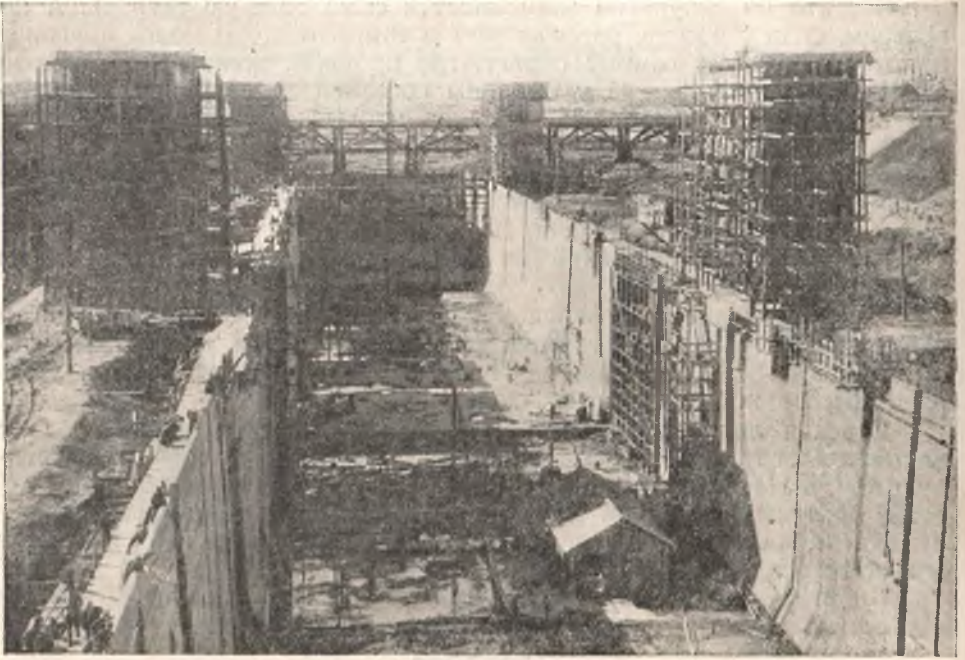
На стройке канала Москва—Волга. Рабочие заканчивают бетонировку шлюза. Шлюз так велик, что большой сарай, стоящий на железобетонном дне шлюза, кажется крошечной избушкой.
