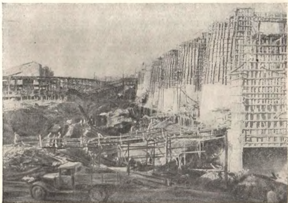
На стройке канала Москва—Волга. Сооружение гигантской железобетонной Волжской плотины.
