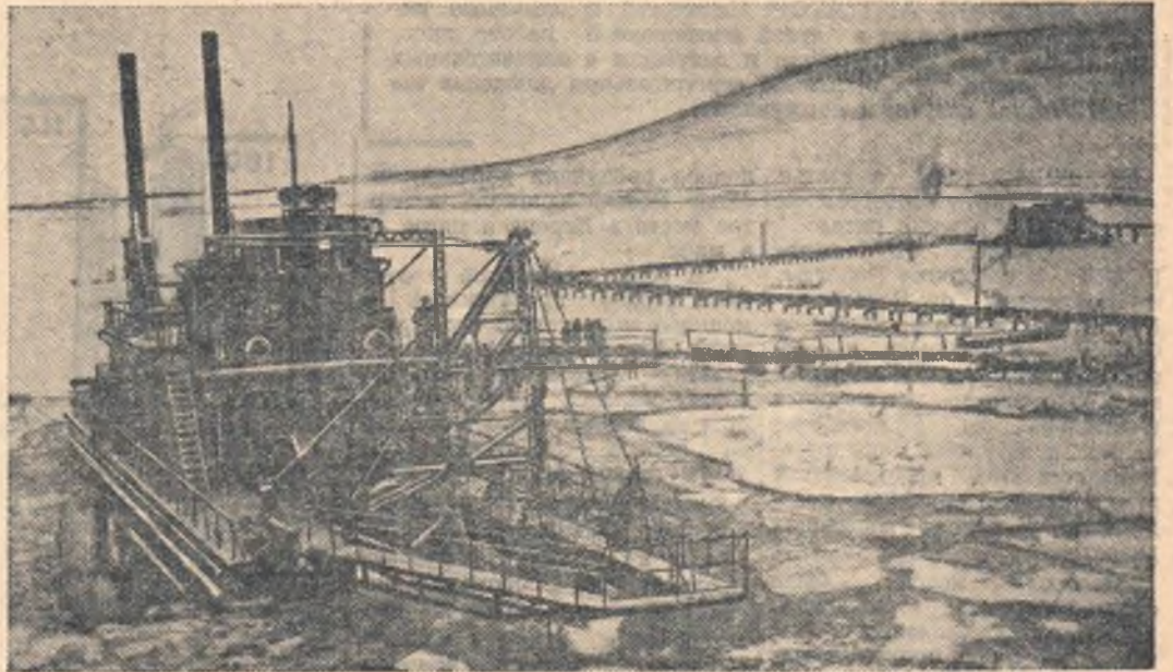
КУЙБЫШЕВГИДРОСТРОИ. Земснаряд № 319 в зимних условиях ведет намыв грунта в перемышку котлована под здание ГЭС. Экипаж намывает 5.000 кубометров грунта вместо 1.200 кубометров по норме. Фото М. Клименкова (Фотохроника ТАСС).
