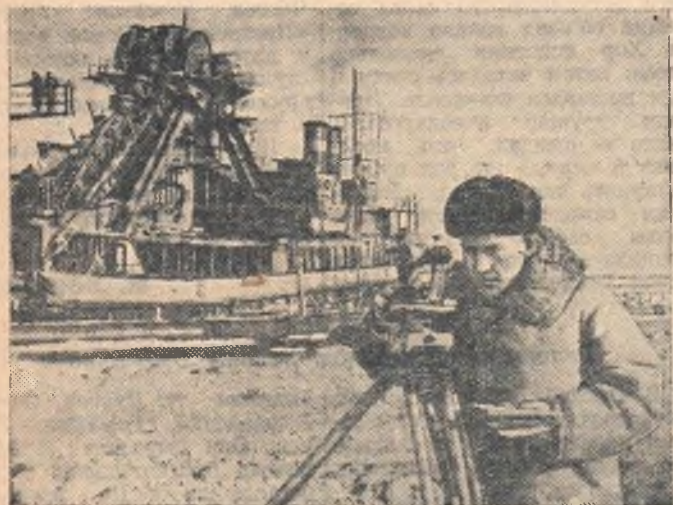
КУЙБЫШЕВГИДРОСТРОЙ. Строительство перемычки котлована ГЭС. Техник-геодезист комсомолец К. Э. Тусинов разбивает площадку для забивки шпунта. Фото М. Клименкова (Фотохроника ТАСС).
