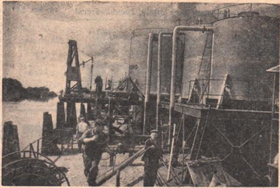
На днях из затона омского судоремонтного завода имени Сталина отправится в путь первая заправочная база. Теперь суда смогут прямо на ходу заправляться горючим, смазочными маслами. НА СНИМКЕ: онончателная проверка всех агрегатов заправочной базы. Фото Э. Савина.
