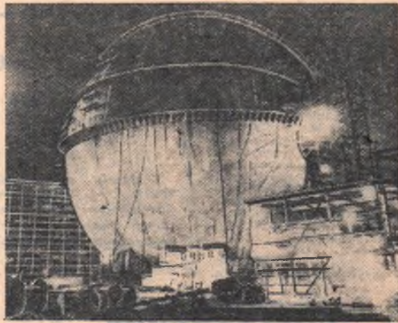
На строительстве атомного реактора в научно-исследовательском центре в Даунри (Шотландия). Диаметр этого герметически закрытого шара, в котором разместится реактор, превышает диаметр купола знаменитого собора святого Павла в Лондоне.
